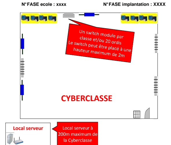
Grande école primaire (Plan E)
