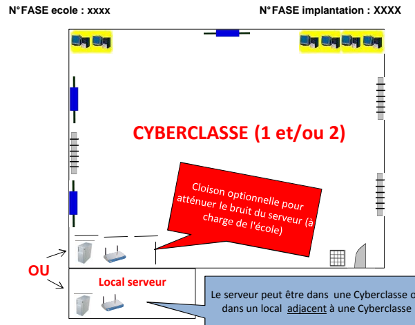
Petite école avec un local serveur ou avec le serveur dans la cyberclasse (Plan D)
