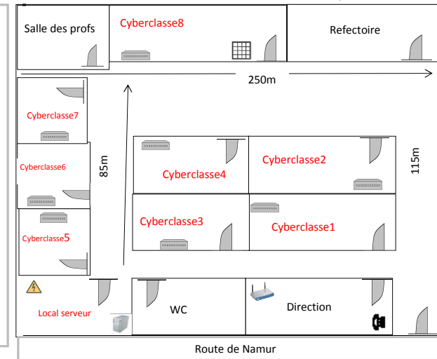
Petite école avec un local serveur ou avec le serveur dans la cyberclasse (Plan D)
