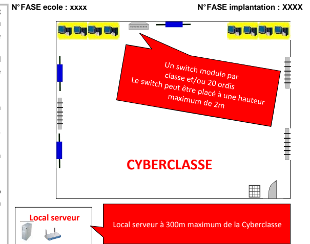
Grande école secondaire (Plan I)
