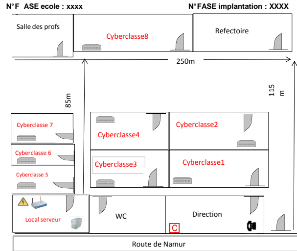
Plan global grande école secondaire (plan H) (option 8 locaux) (+ 90 élèves)
